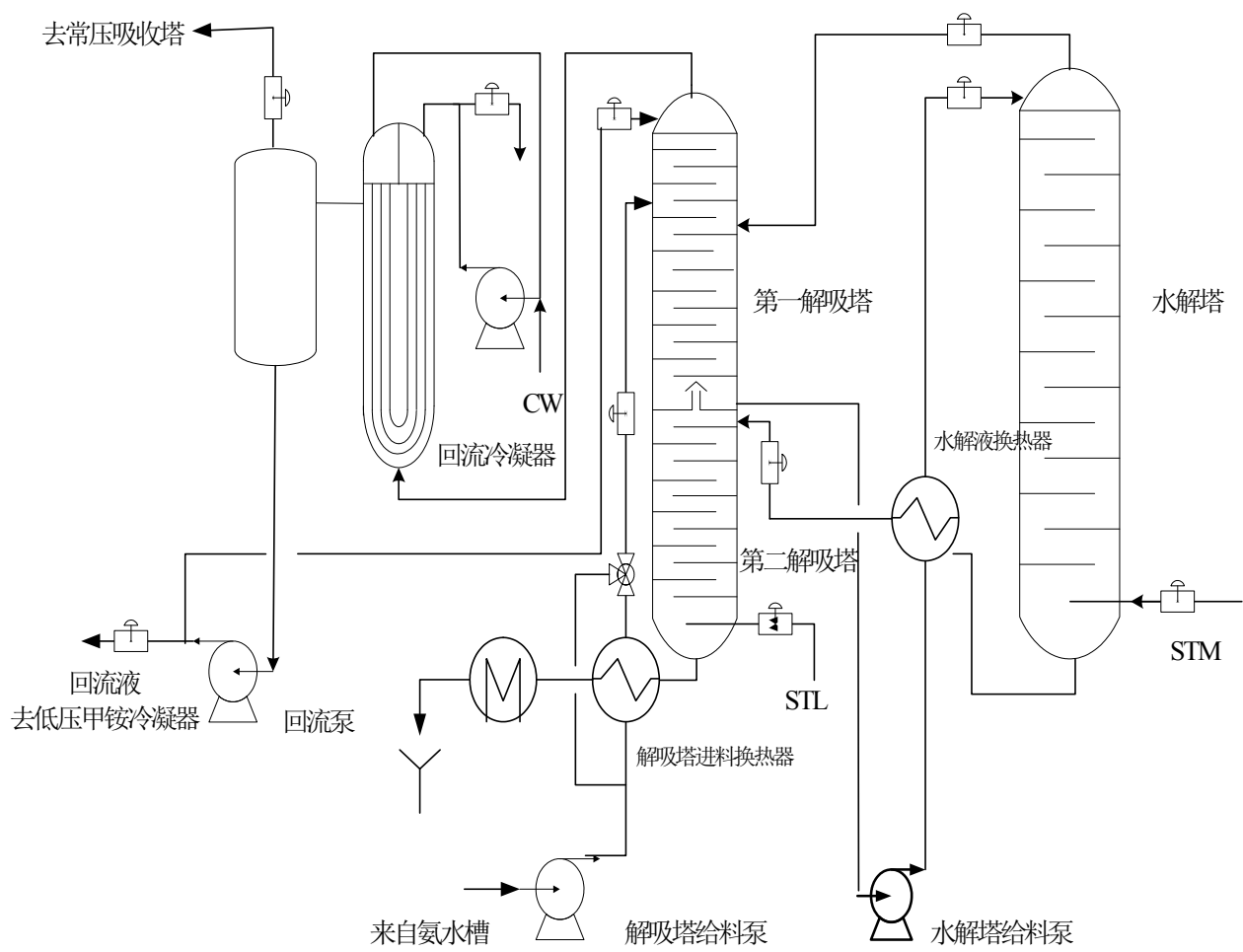
图 3-7 Stamicarbon 高温水解流程
